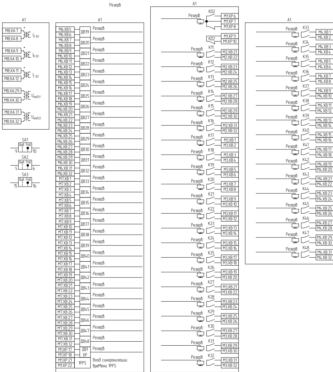
Рисунок В.3 – Схема электрическая принципиальная (часть 3)
